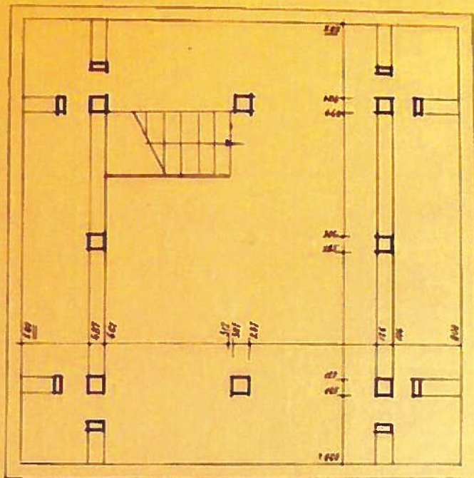
II AUKŠTO PLANAS
